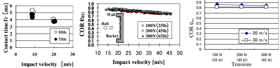
図3 接触時間、テンション、衝突速度、反発係数の関係（実測例）（川副2003、Kawazoe ら2003）
