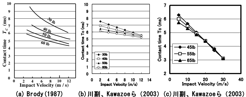
図2 接触時間、テンション、衝突速度の関係
